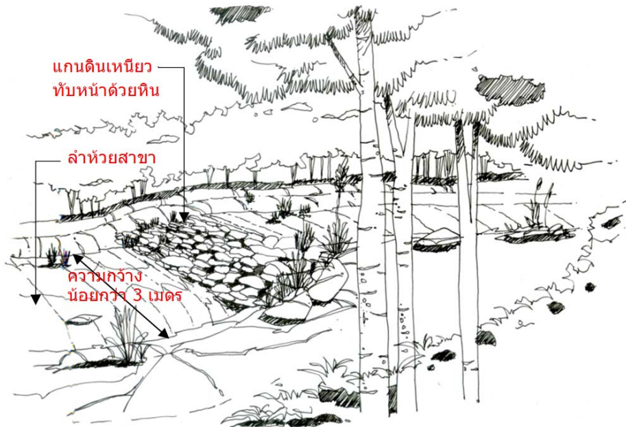
ฝายดินเหนียว
